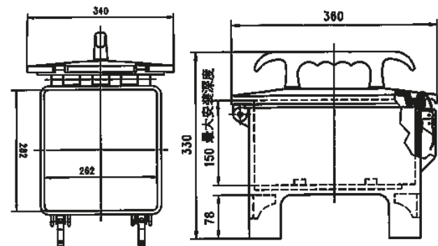
图纸 5 MB 43 尺寸毫米
