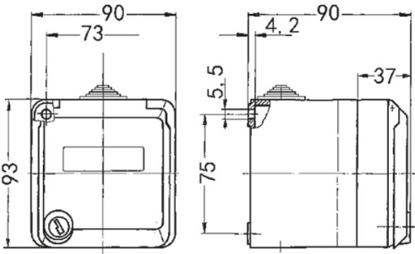
图纸 1 MB 564 尺寸毫米
