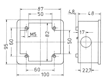
图纸 1 MB 232 尺寸毫米
