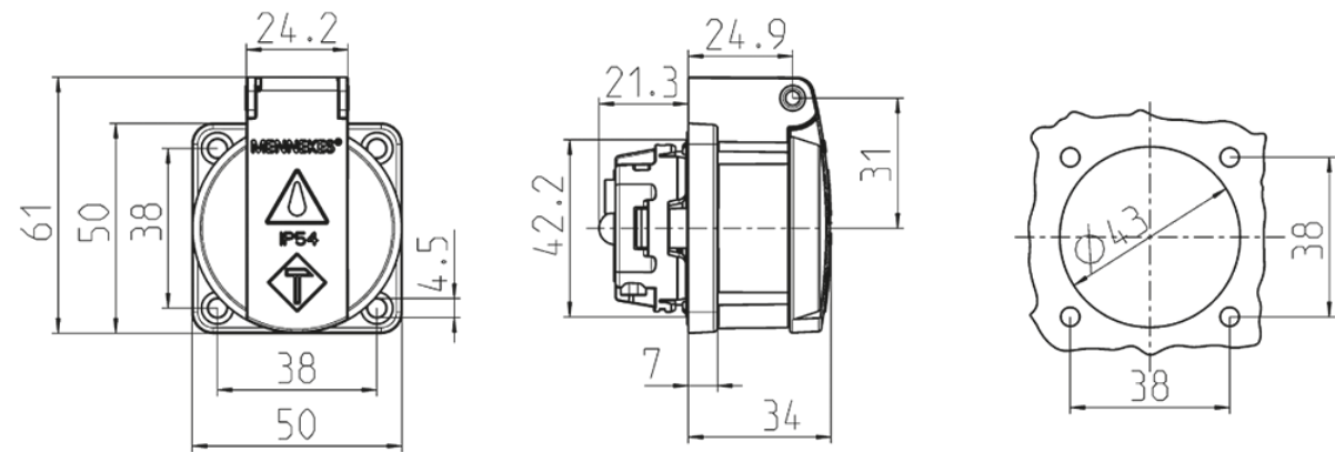
图纸 1 MB 5861 尺寸毫米
